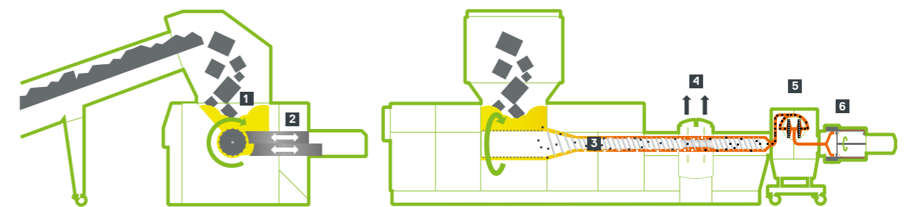
1 Triturador mono-rotor 2 Sistema de doble empujador 3 Extrusora configurada coaxialmente 4 Zona de desgasificación 5 Filtro automático y autolimpiable 6 Sistema granceador
